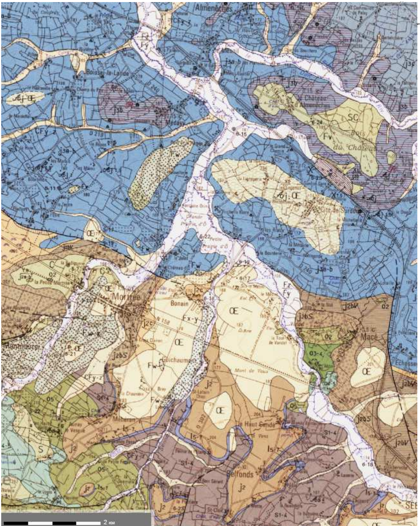
Carte géologique - Sées (n°213)
